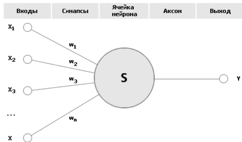
Рис. 1. Искусственный нейрон
