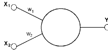
Рис. 4. Однонеуронный перцептрон
